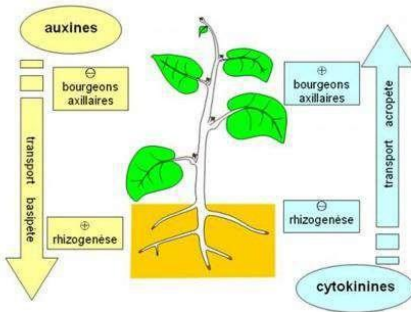
Figure 2 la balance hormonale de la plante in vitro
