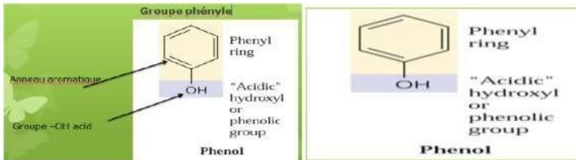
Figure 24 Le groupe phénol chez les Molécules Phénoliques
