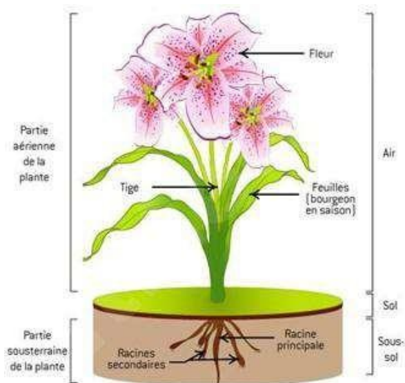
Figure 1 le matériel végétal d'une plante
