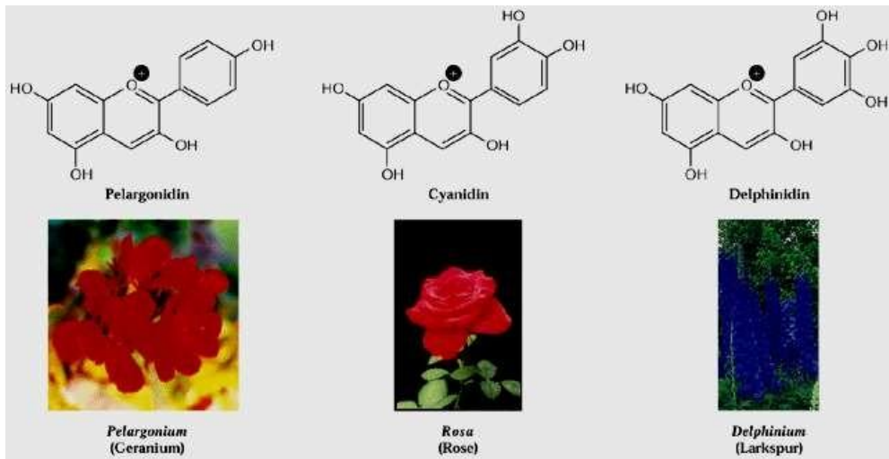
Figure 26 structure de flavonoïdes
