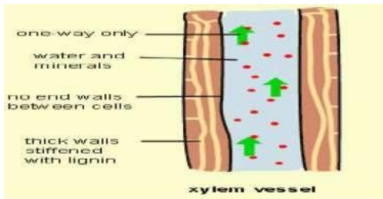
Figure 25 Lignine des parois végétales
